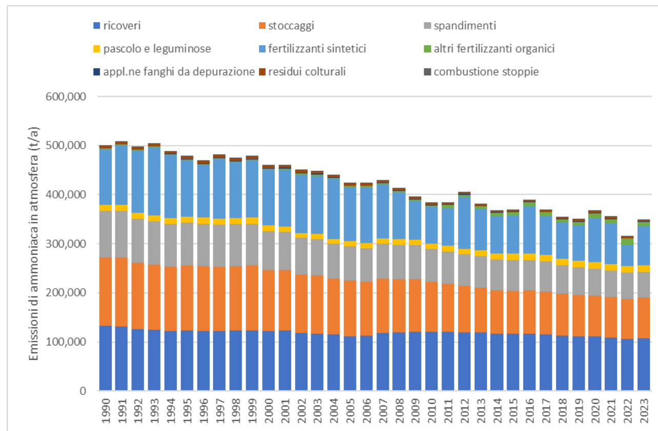
Emissioni di ammoniacale per fonte di emissione (v.a.) (1990-2023)
