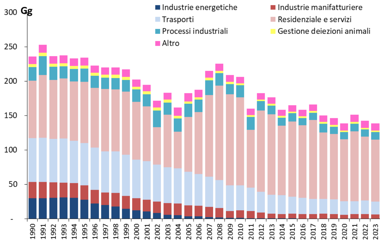
Serie storica 1990-2023 delle emissioni di polveri sottili \leq 2.5\mu\text{m} (Gg)
