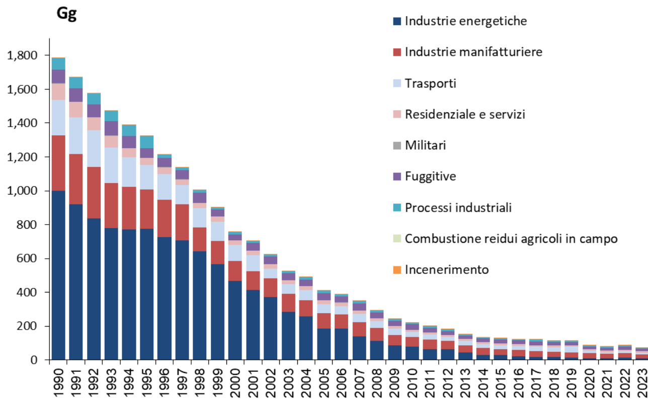
Serie storica 1990-2023 delle emissioni di ossidi di zolfo (SO x ) (Gg)
