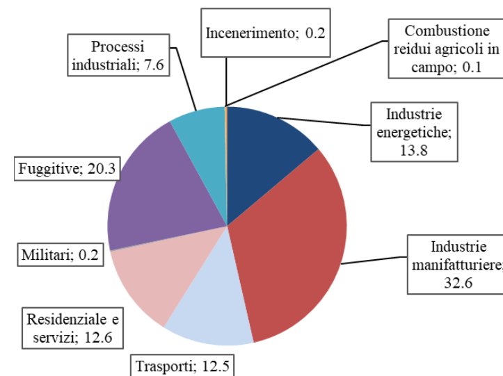
Ripartizione percentuale emissioni di SO x per settore - 2023
