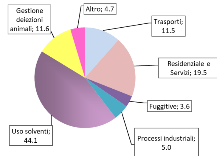
Ripartizione percentuale emissioni di COVNM per settore - 2023
