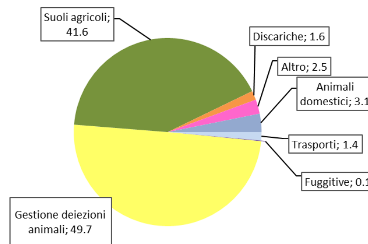
Ripartizione percentuale emissioni di \text{NH}_3 per settore - 2023
