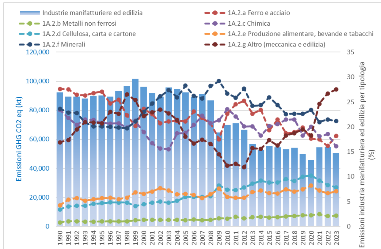
Emissioni di gas serra CO 2 eq. del settore industrie manifatturiere ed edilizia e ripartizione percentuale per tipologia (1990-2023)
