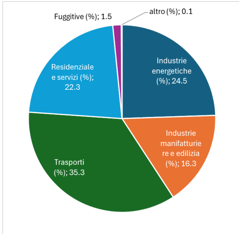
Ripartizione percentuale delle emissioni di gas serra per tipologia (2023)
