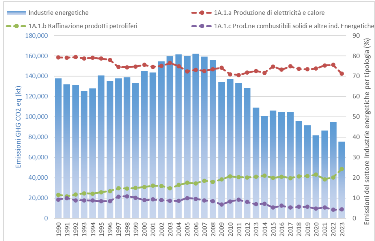
Emissioni di gas serra CO 2 eq. del settore industrie energetiche e ripartizione percentuale per tipologia (1990-2023)
