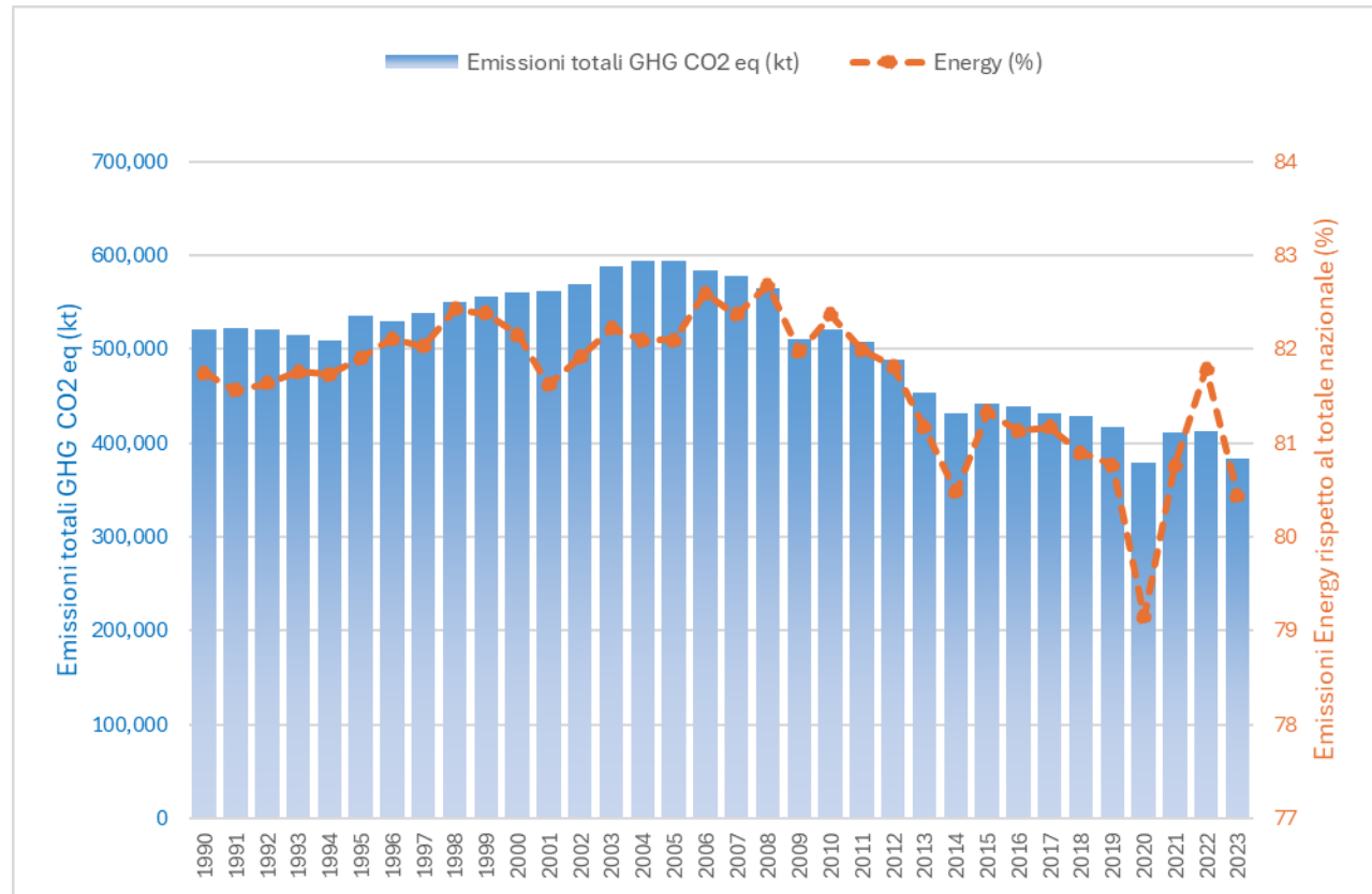
Emissioni di gas serra CO 2 eq (kt) e contributo del settore energetico al totale nazionale (1990-2023)
