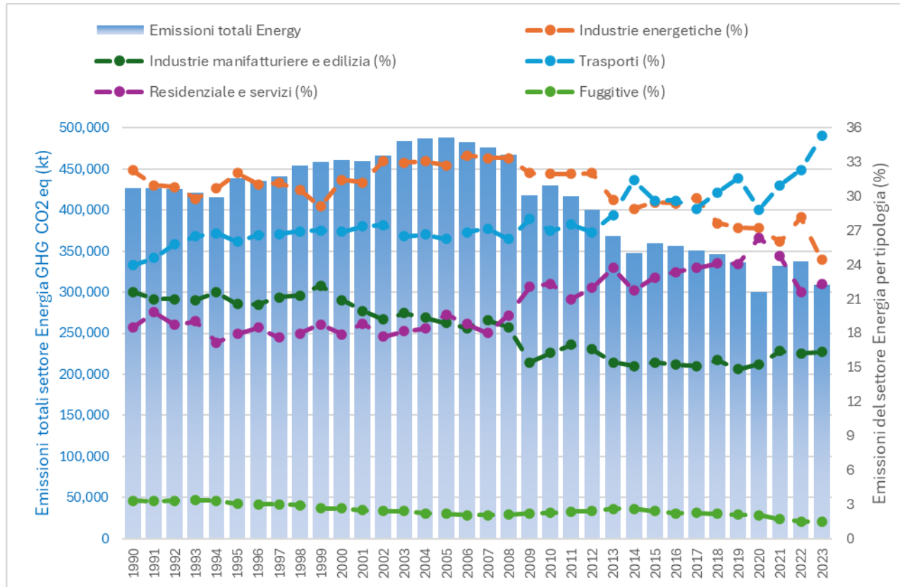
Emissioni di gas serra CO 2 eq (kt) del settore energetico e ripartizione percentuale per tipologia (1990-2023)
