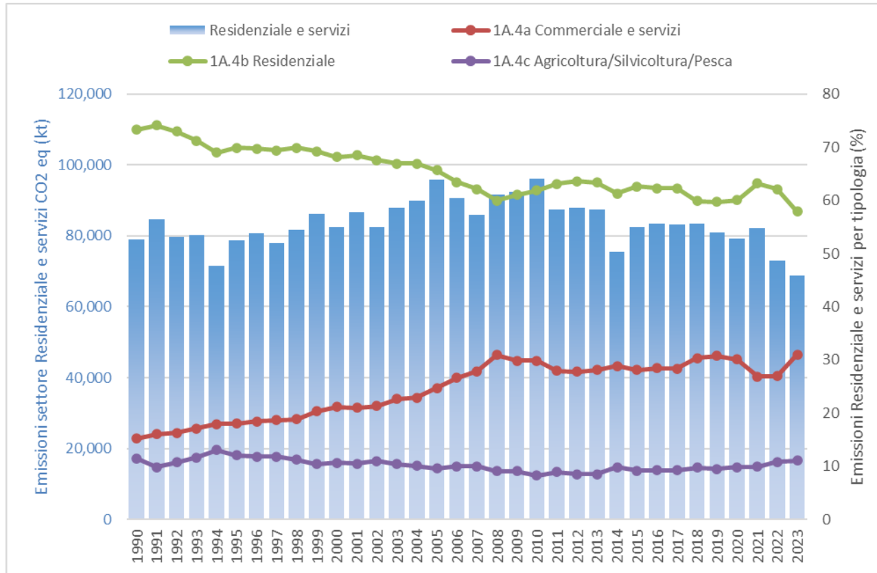
Emissioni di gas serra CO 2 eq (kt) del settore residenziale e servizi e ripartizione percentuale per tipologia (1990-2023)
