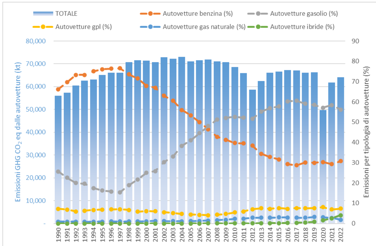
Emissioni di gas serra dalle autovetture per tipologia di alimentazione in Italia dal 1990 al 2022
