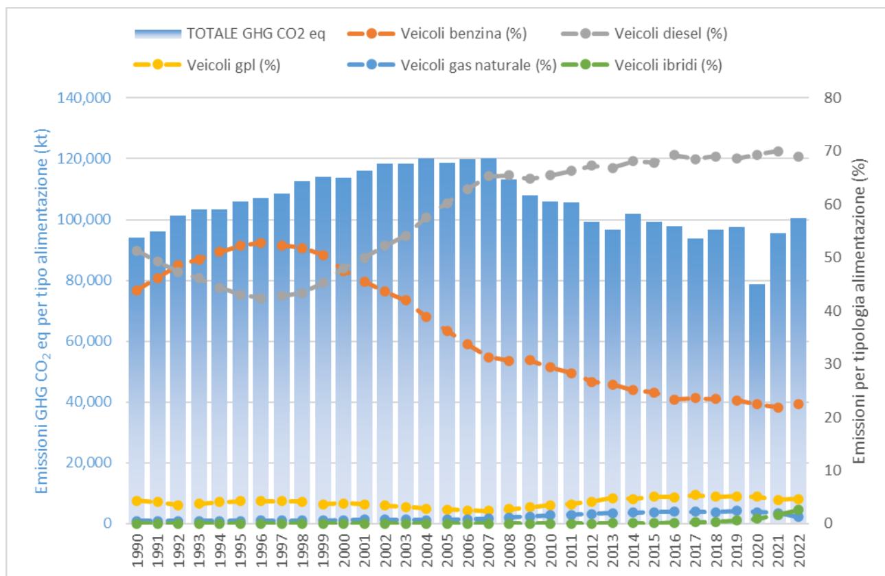
Emissioni di gas serra per tipologia di alimentazione (1990-2022)
