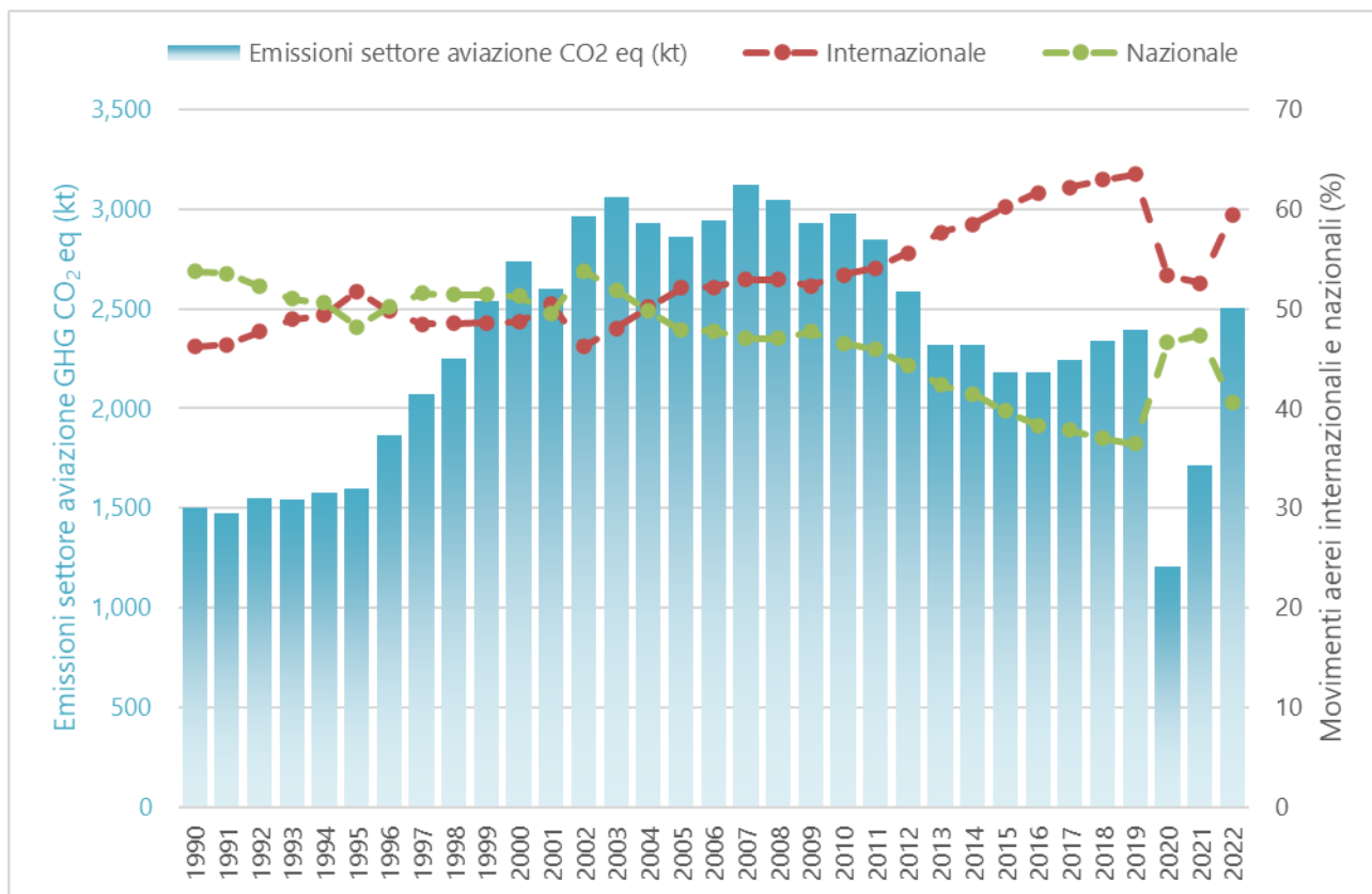
Emissioni di gas serra e consumi di carburanti dell'aviazione (1990-2022)
