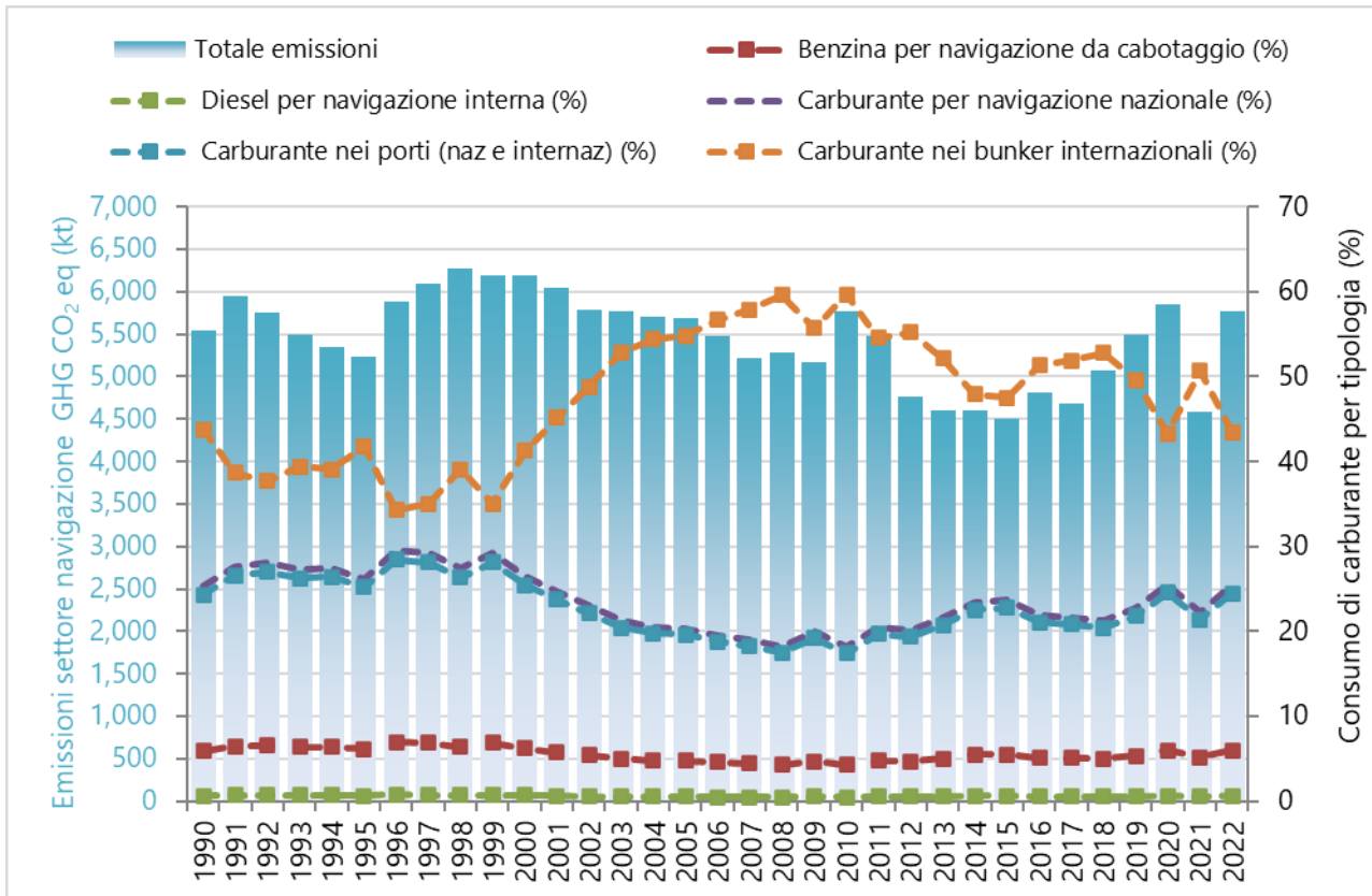
Emissioni di gas serra e consumi di carburanti della navigazione (1990-2022)
