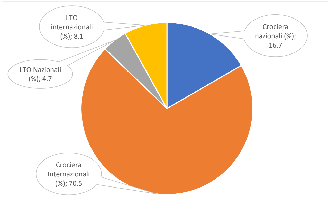
Ripartizione dei consumi di carburanti per le fasi di volo (valori percentuali) – anno 2022
